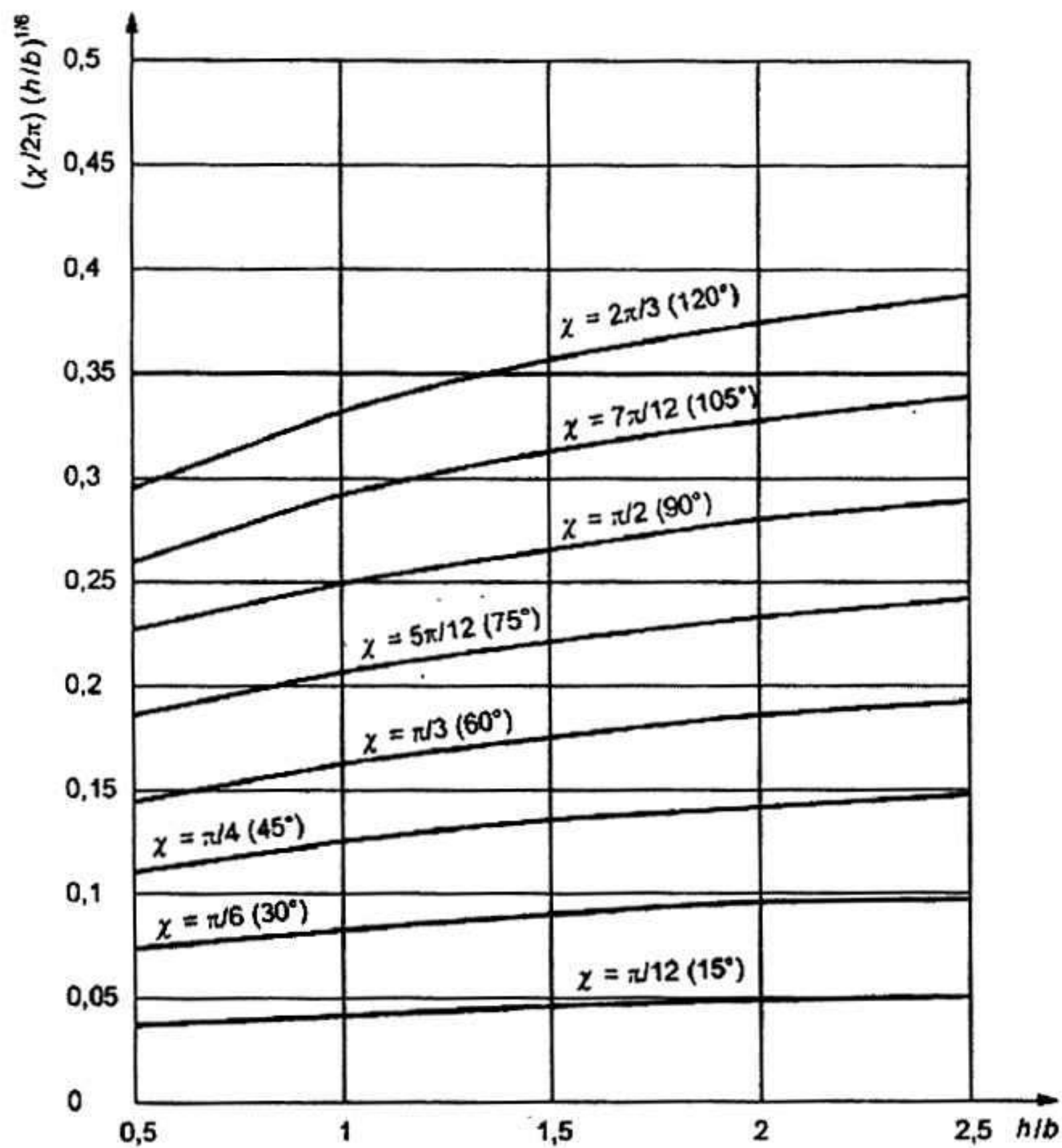
Hình D.2 – Biểu đồ của (X/2\pi)(h/b)^{1/6} đối với h/b dùng cho tính toán tổn thất áp suất trong ống khuỷu ở đầu ra
