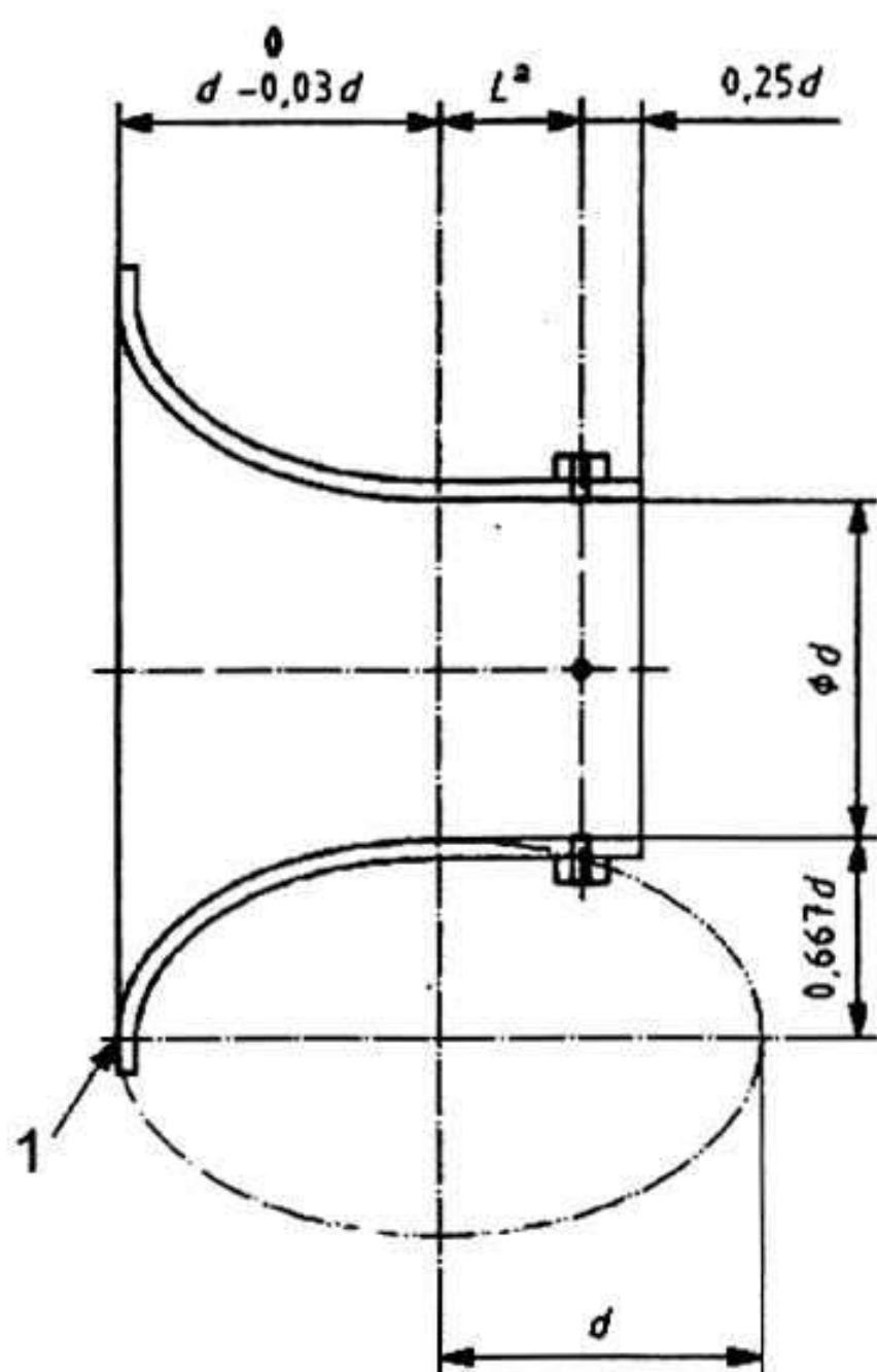
a) Vòi (miệng) phụ có các đầu nổi ở cổ
