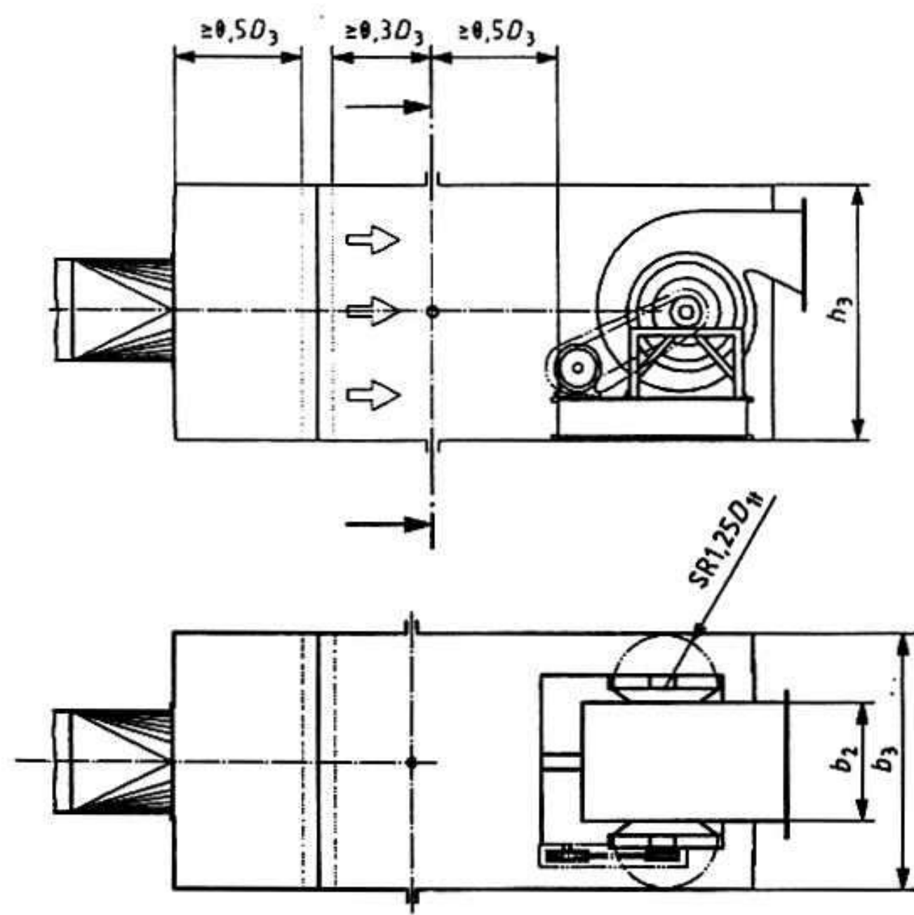
c) Các kích thước nhỏ nhất của buồng thử kéo dài dùng cho lắp đặt các quạt có đầu vào kép. Hình 37 – Buồng thử kiểu 2 ở phía đầu vào (tiếp theo)
